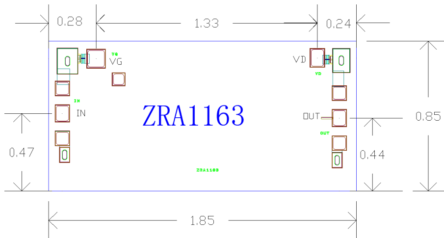
Figure 2. 外形尺寸
