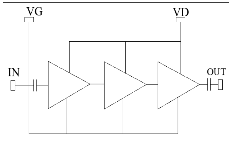
Figure 1. 管脚信息
