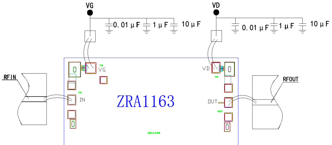
Figure 3. 装配示意图
